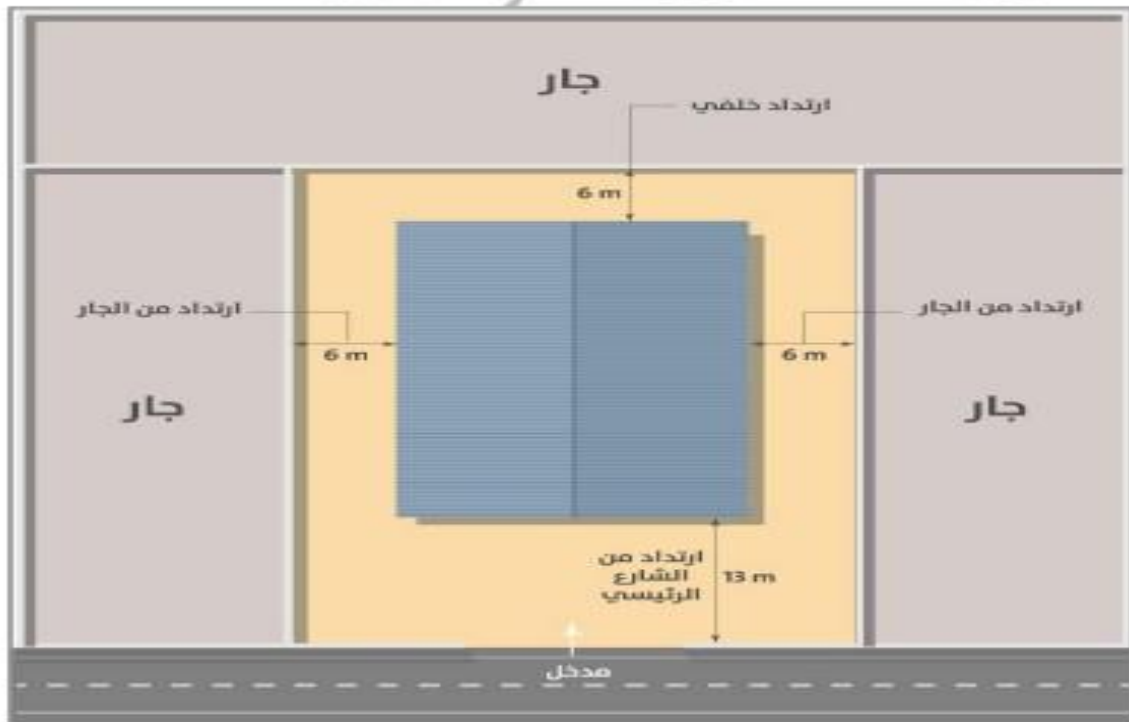
مثال (ب) يوضح الارتدادات في المواقع المعتمدة كمخططات للمواقع
